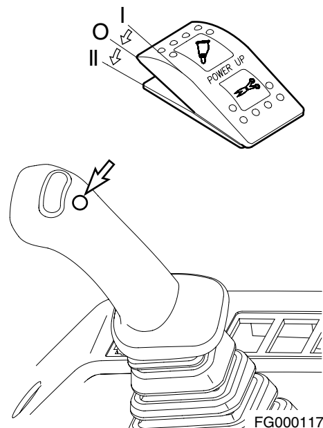
Figura 43 PALANCA DE MANDO DERECHA (JOYSTICK)
